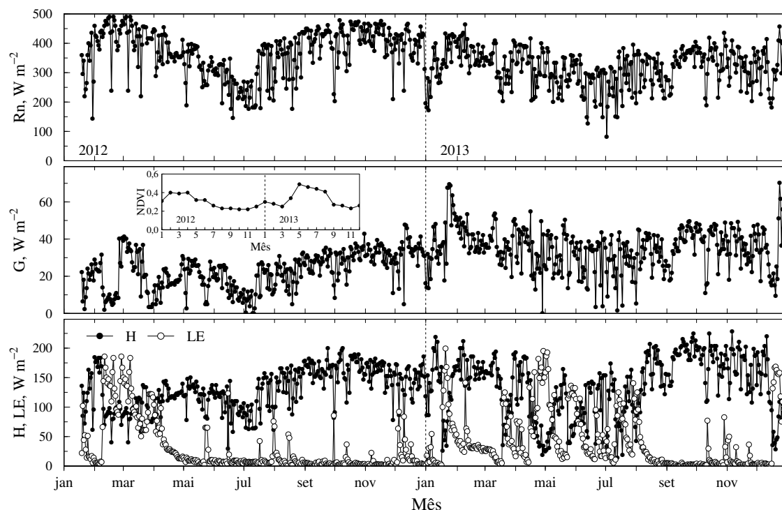
Figura 9. Variação sazonal dos fluxos de energia (saldo de radiação, R_n , e fluxos de calor latente, LE, sensível, H, e no solo, G) em área cultivada com pastagem durante os anos de 2012 e 2013 em Serra Talhada, PE.
