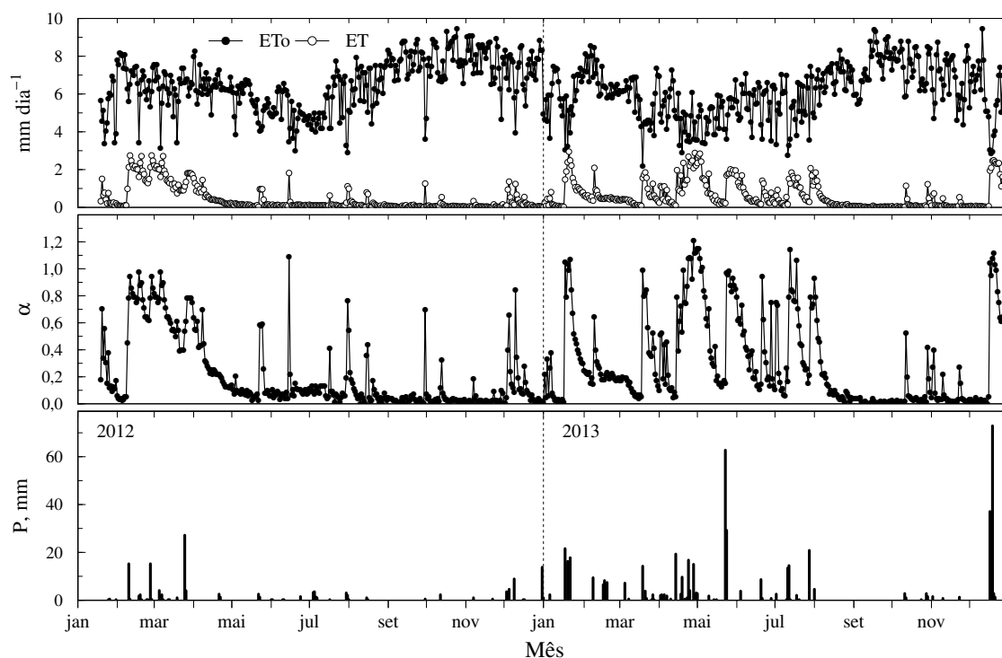
Figura 11. Variação sazonal da evapotranspiração (ET), evapotranspiração de referência (ET o ), constante de Priestley-Taylor ( \alpha ) e a precipitação pluviométrica (P) em pastagem.
